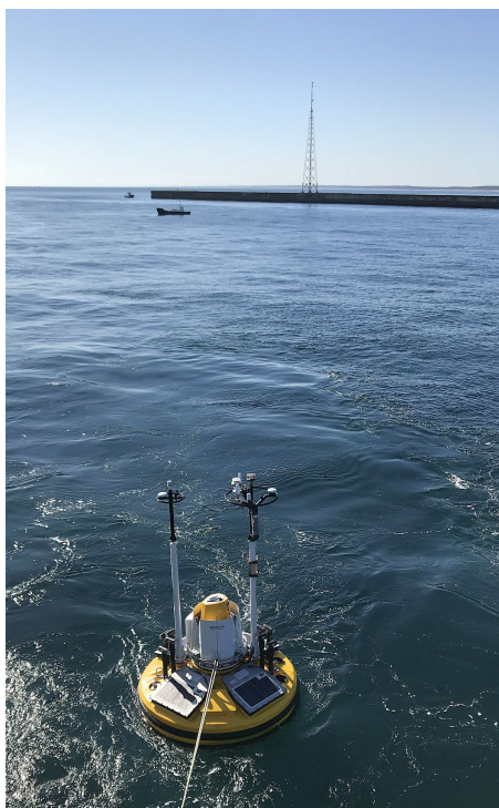
青森県むつ小川原港におけるフローティングライダー観測 (2019-21年度 NEDOF「洋上風況調査手法の確立」事業)
